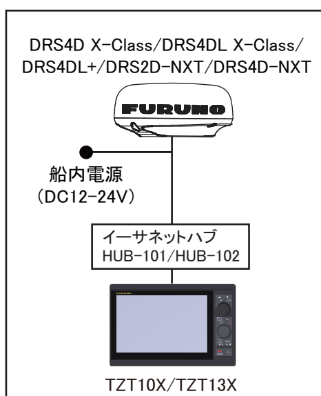
レーダーセンサー(レドームタイプ)接続例
