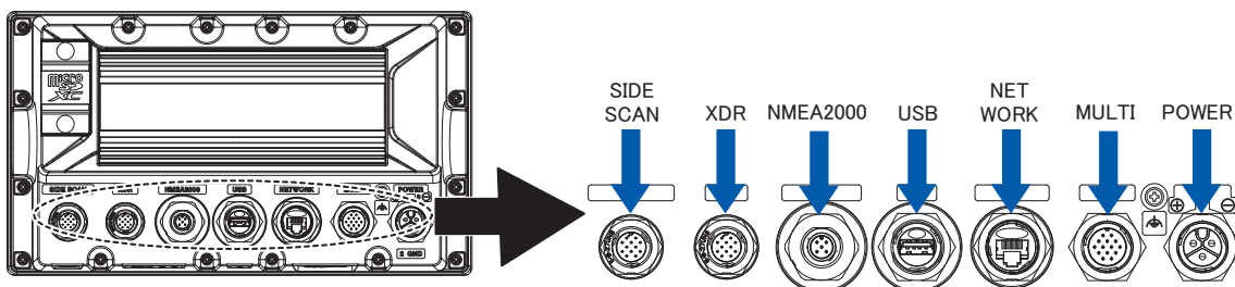
機器背面
