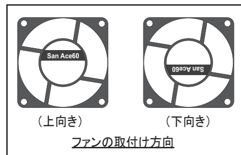
FAN3 (下向きに取付け)
