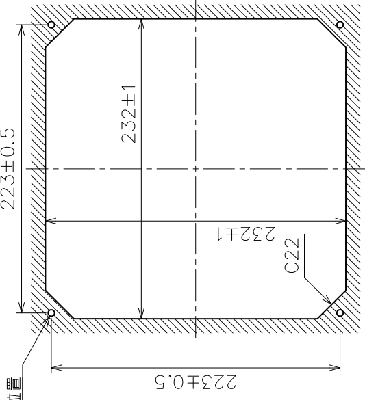
取付穴寸法 CUTOUT DIMENSIONS
